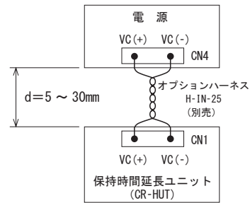
図6.10 接続方法
