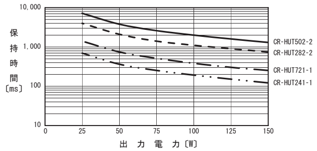
図6.11 LHA150F-□-U1 保持時間-出力電力特性 (参考値)
