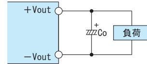
図6.13 出力側外付けコンデンサ接続方法
