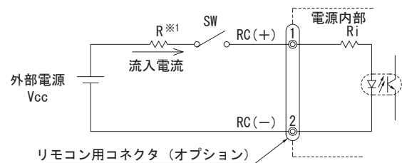
図6.2 リモートコントロール使用例
