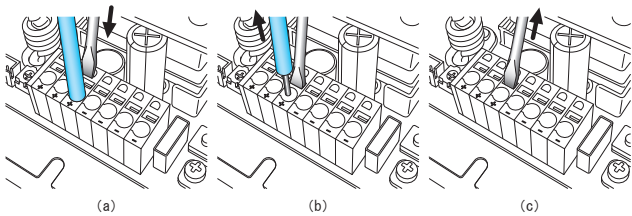
図6.7 フェール端子、単線、撚線の解除概略図
